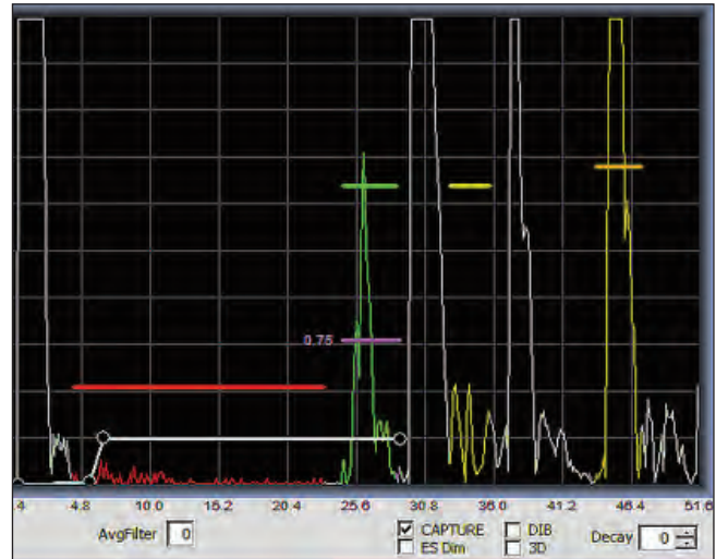
图为UT界面的A-扫描显示，图示通道1设置了1个界面闸门和4个测量闸门
