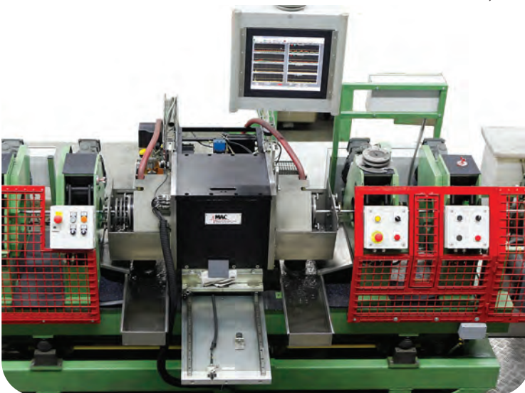
图为Echomac®仪器以及Echomac®旋转体，用于检测不锈钢和钛合金热交换管
